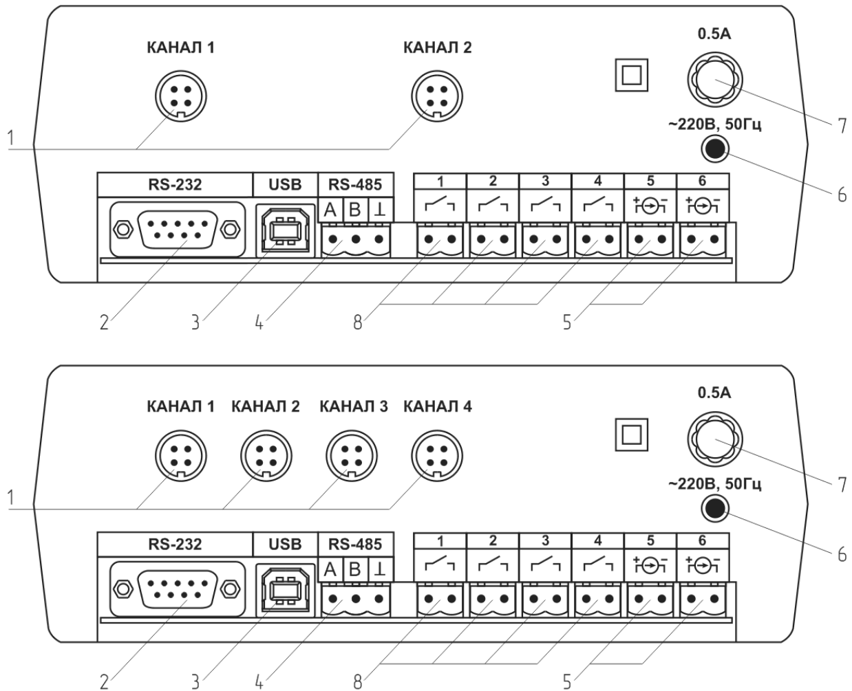
Рисунок 3.2 Задняя панель прибора сверху вниз: ИВТМ-7 /2-С-4Р-2А, ИВТМ-7 /4-С-4Р-2А.
