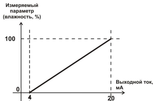
Рисунок 3.14 Линейный выход 4...20 мА по диапазону относительной влажности с границами 0...100%.
