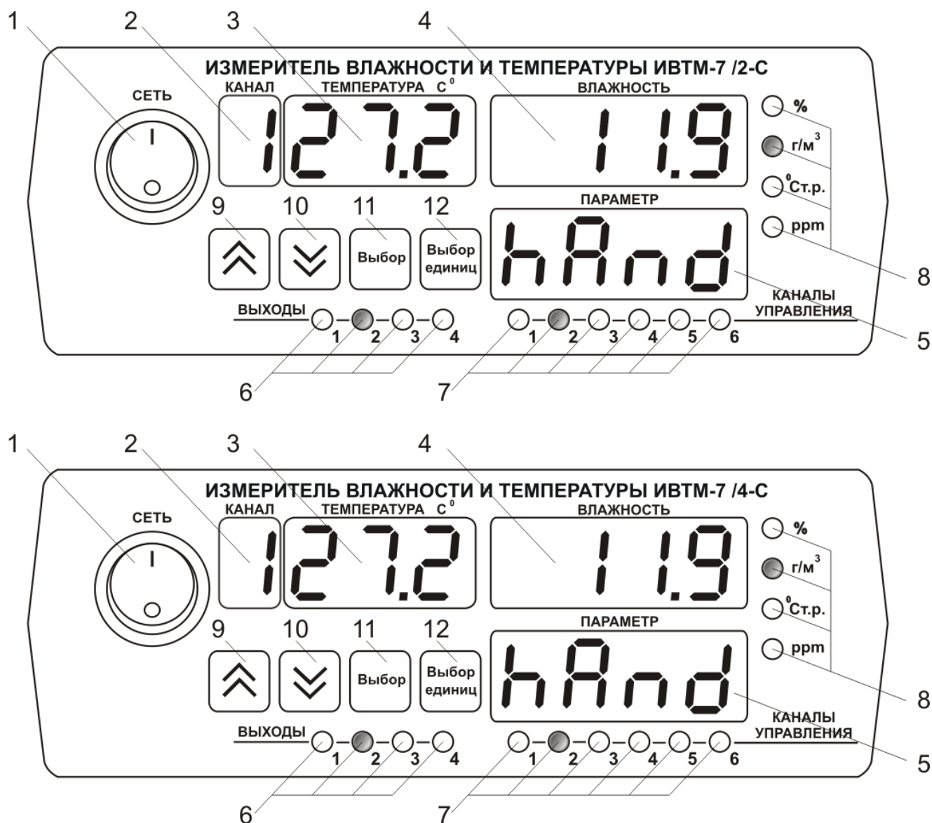
Рисунок 3.1 Вид лицевой панели прибора, исполнение: ИВТМ-7 /2-С-4Р-2А, ИВТМ-7 /4-С-4Р-2А (сверху вниз).
